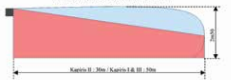
Zona de detección del detector : vista lateral
